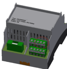
Bornele de alimentare ale expanderului pentru peleți
