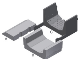
A: blocul (deflectorul), B: camera de ardere din beton refractar, C: arzătorul din inox
